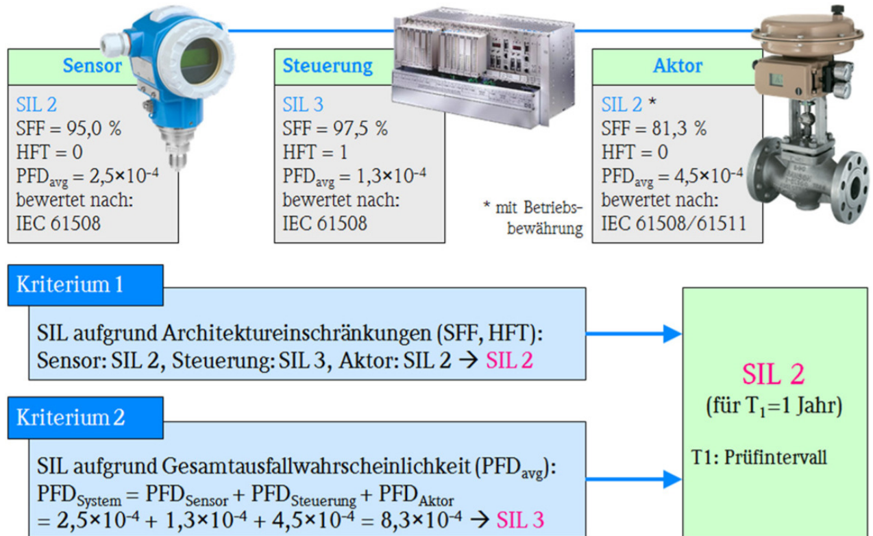
SIL-Nachweis für eine einkanalige PLT-Schutzeinrichtung
