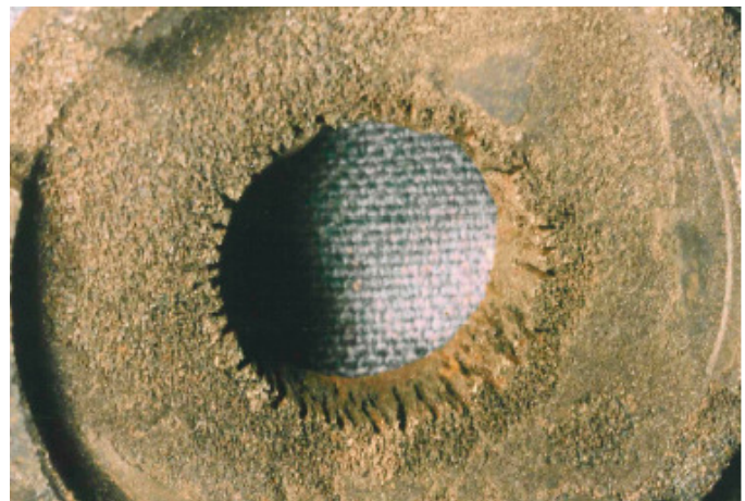
Flashingerosion Sitz
