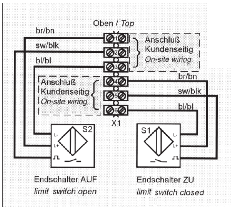
Anschlussschema
