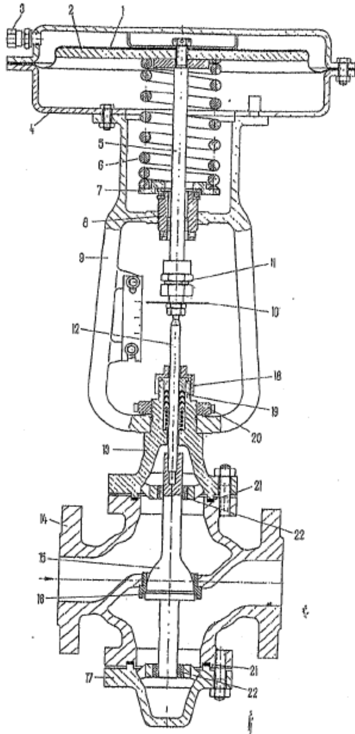
Einsitz-Durchgangsventil, Baureihe 58, zweiseitig geführt, mit pneumatischem, federbelastetem, nichtreversierbarem Stellantrieb
