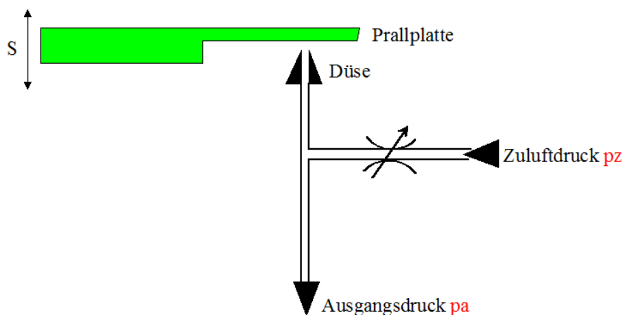
Funktionsprinzip eines Düse-Prallplattensystems
