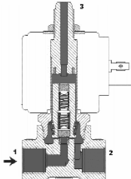
3/2 Wege-Magnetventil „auf“
