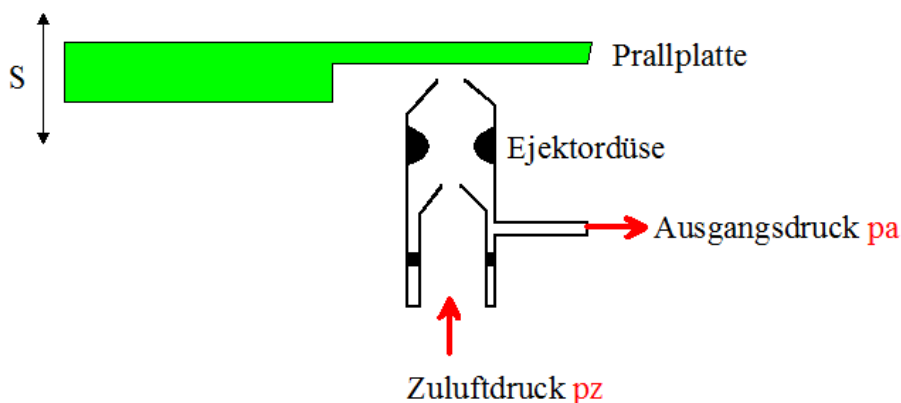
Aufbau einer Ejektoraue
